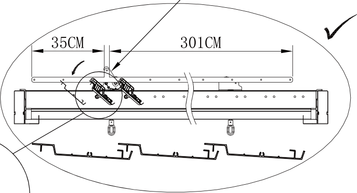
Position de la manivelle
