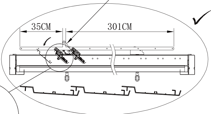
Position de la manivelle
